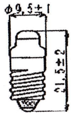
TL9 E10/14
