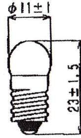
G11 E10/14
