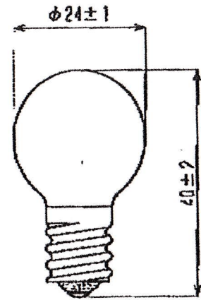
E24 E12/15
