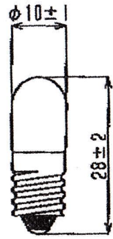
T10 E10/14
