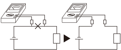
一般電流計の場合
