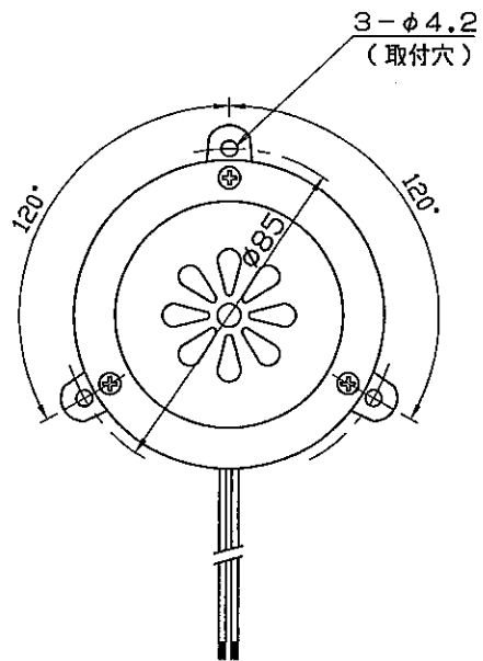
正面図
