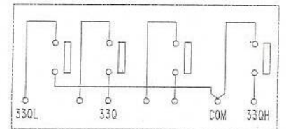
内部接続図
