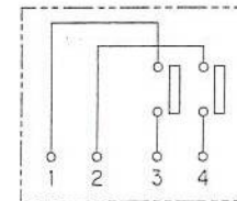
内部接続図
