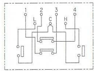
内部接続図
