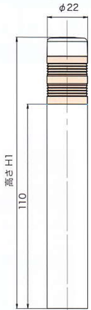
基本寸法図
